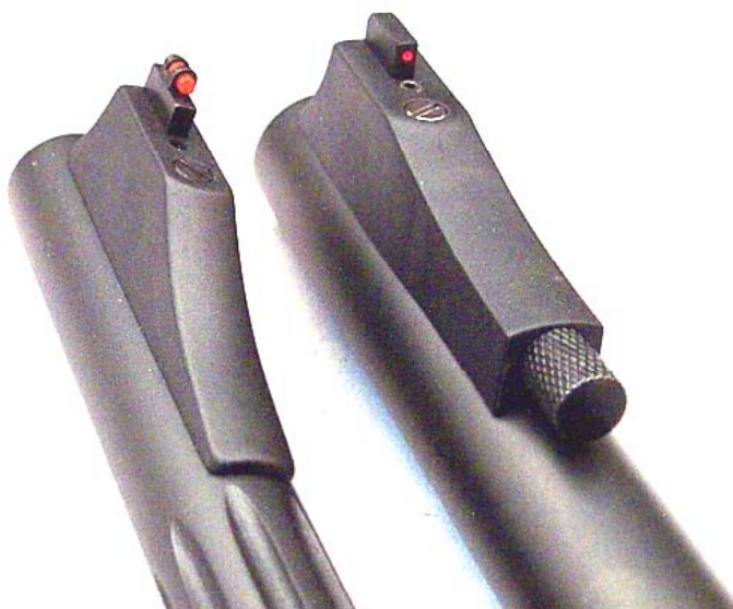
links: konventionelles Leuchtkorn, rechts LED-Leuchtkorn
